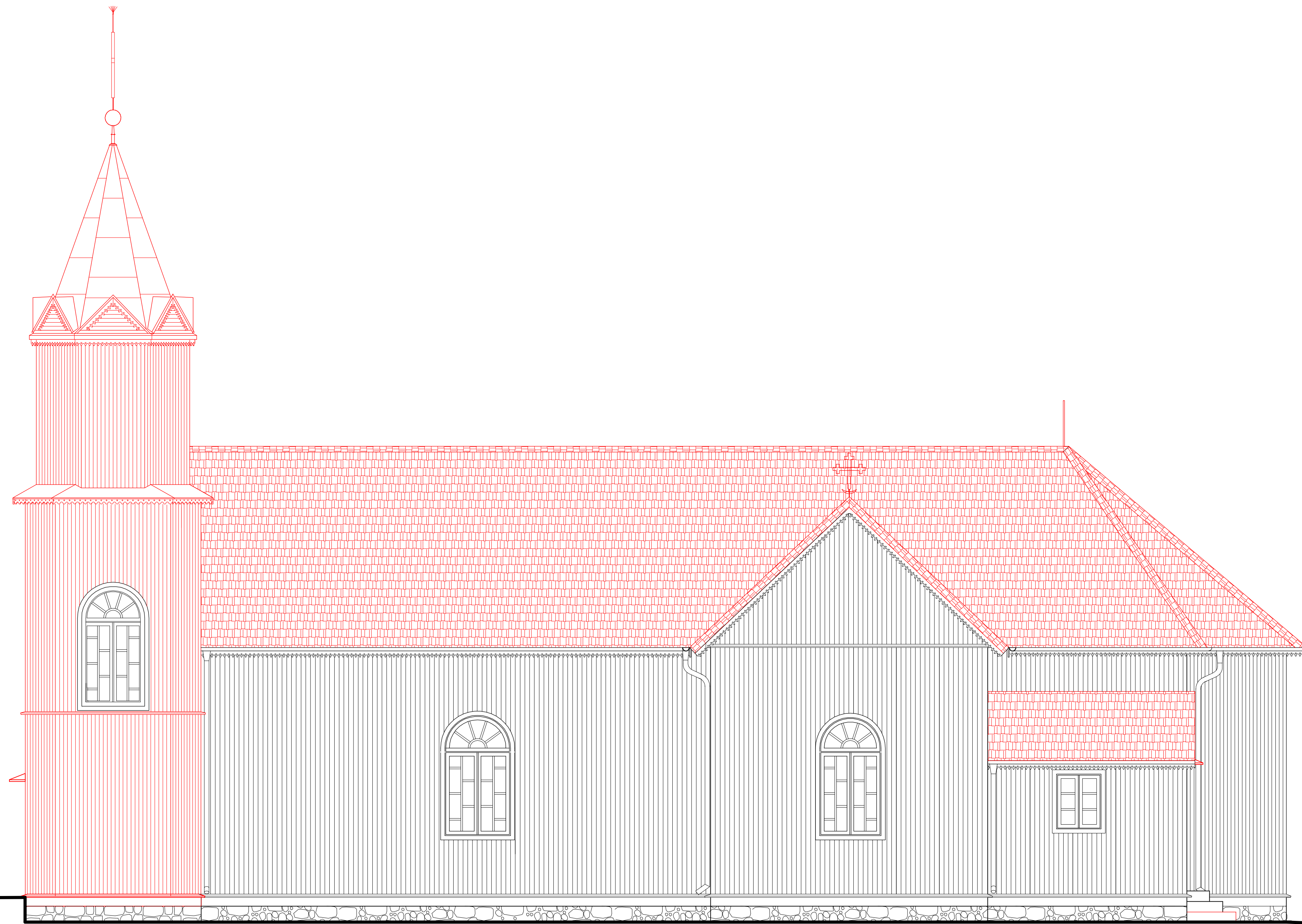
ELEWACJA POŁUDNIOWA 1:50
