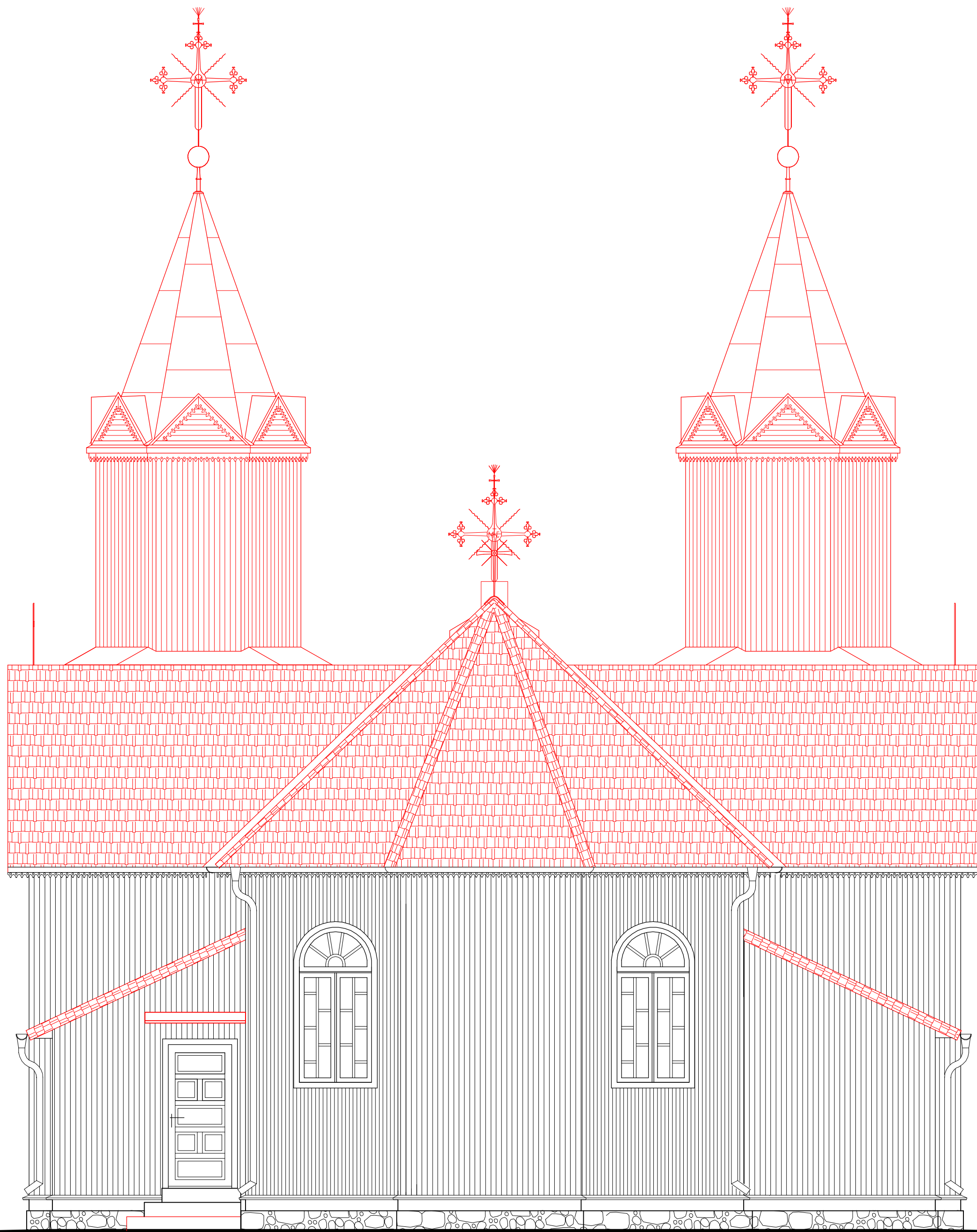
ELEWACJA WSCHODNIA 1:50
