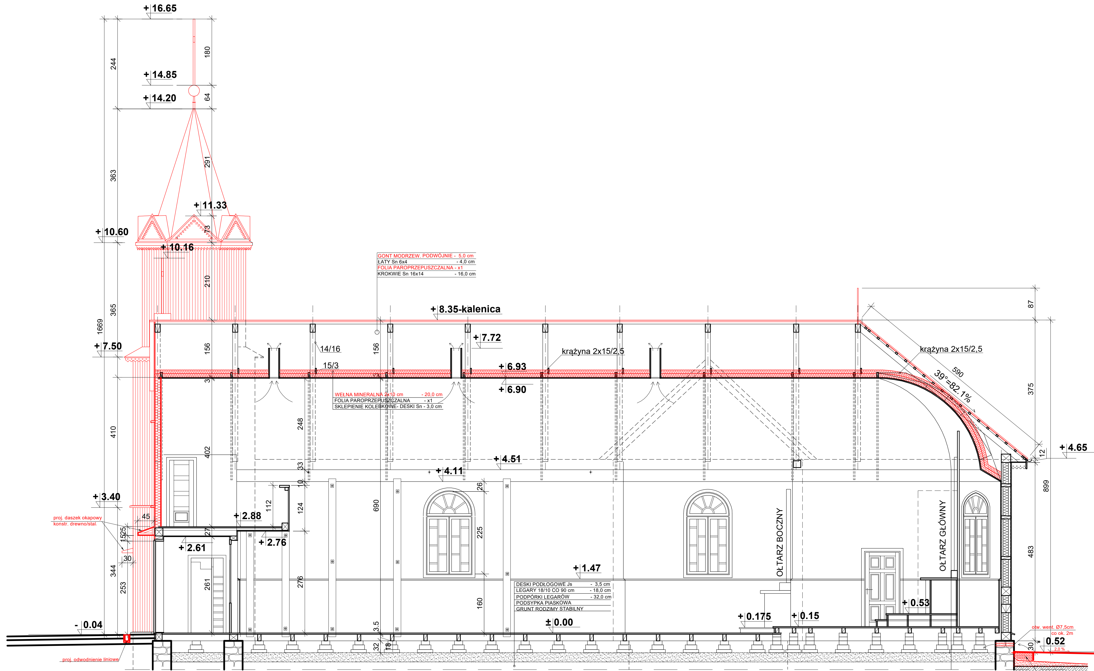
PRZEKRÓJ PIONOWY D-D 1:50
