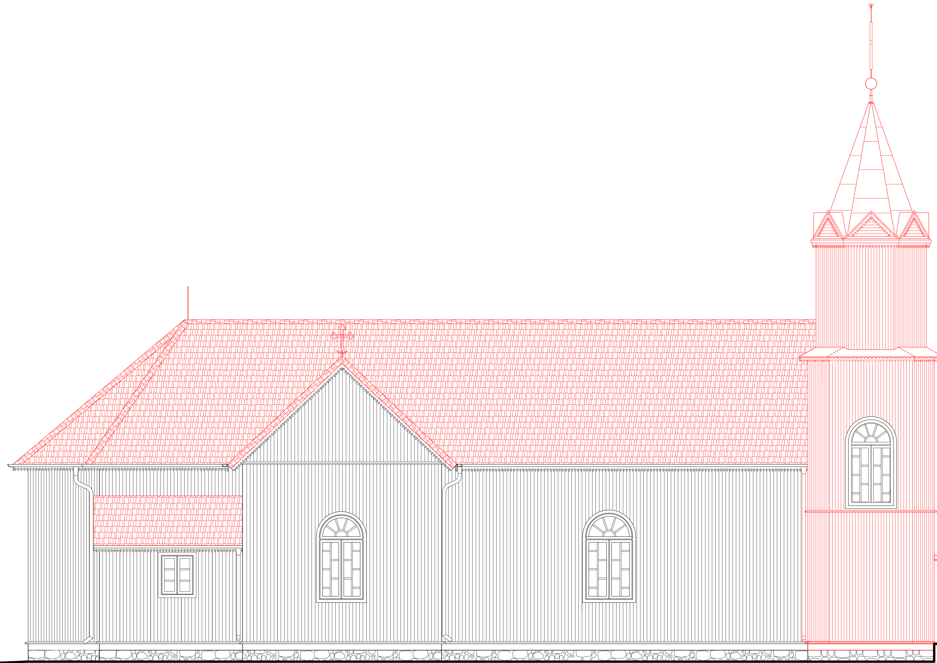
ELEWACJA PÓŁNOCNA 1:50
