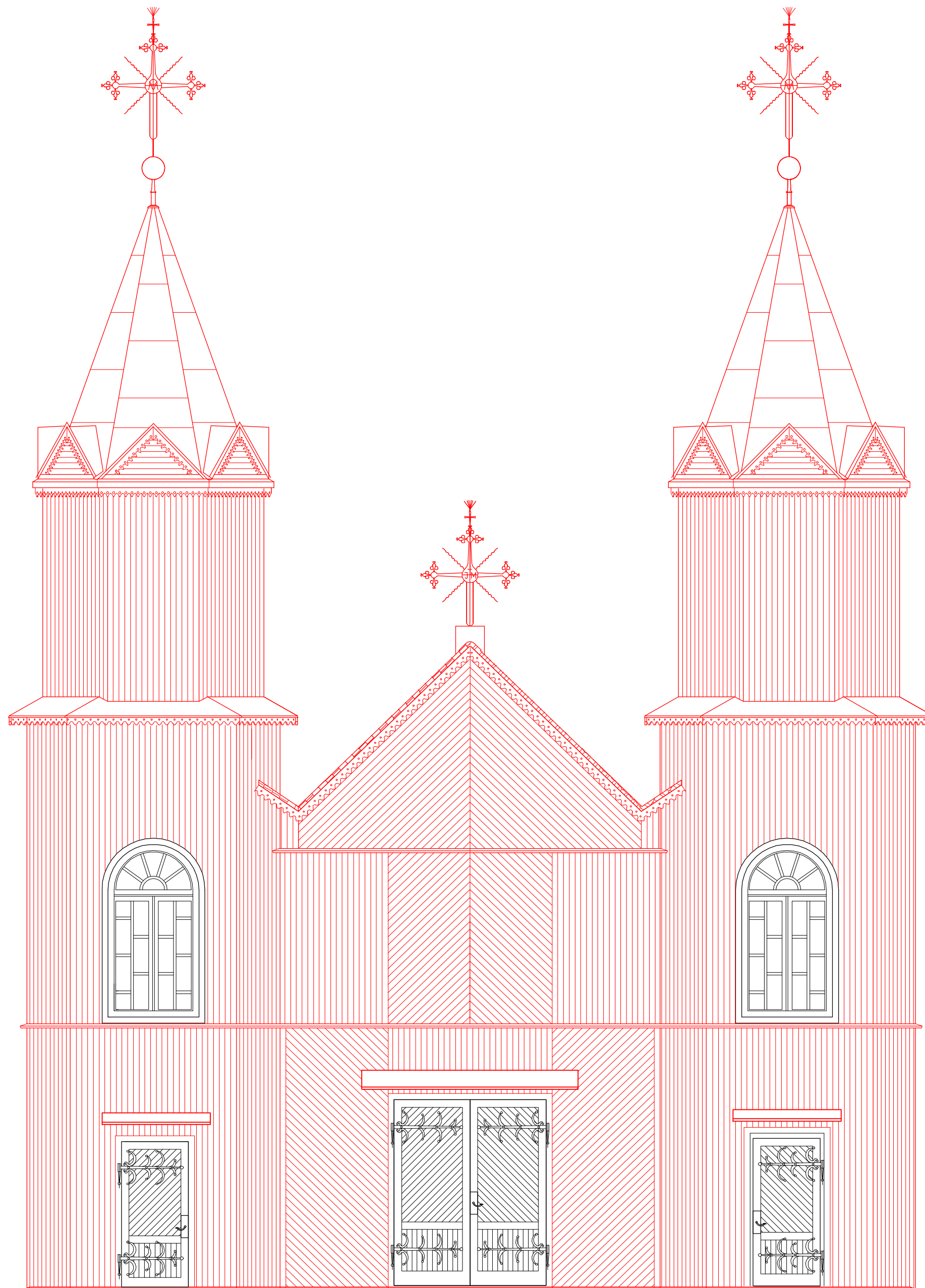
ELEWACJA ZACHODNIA 1:50
