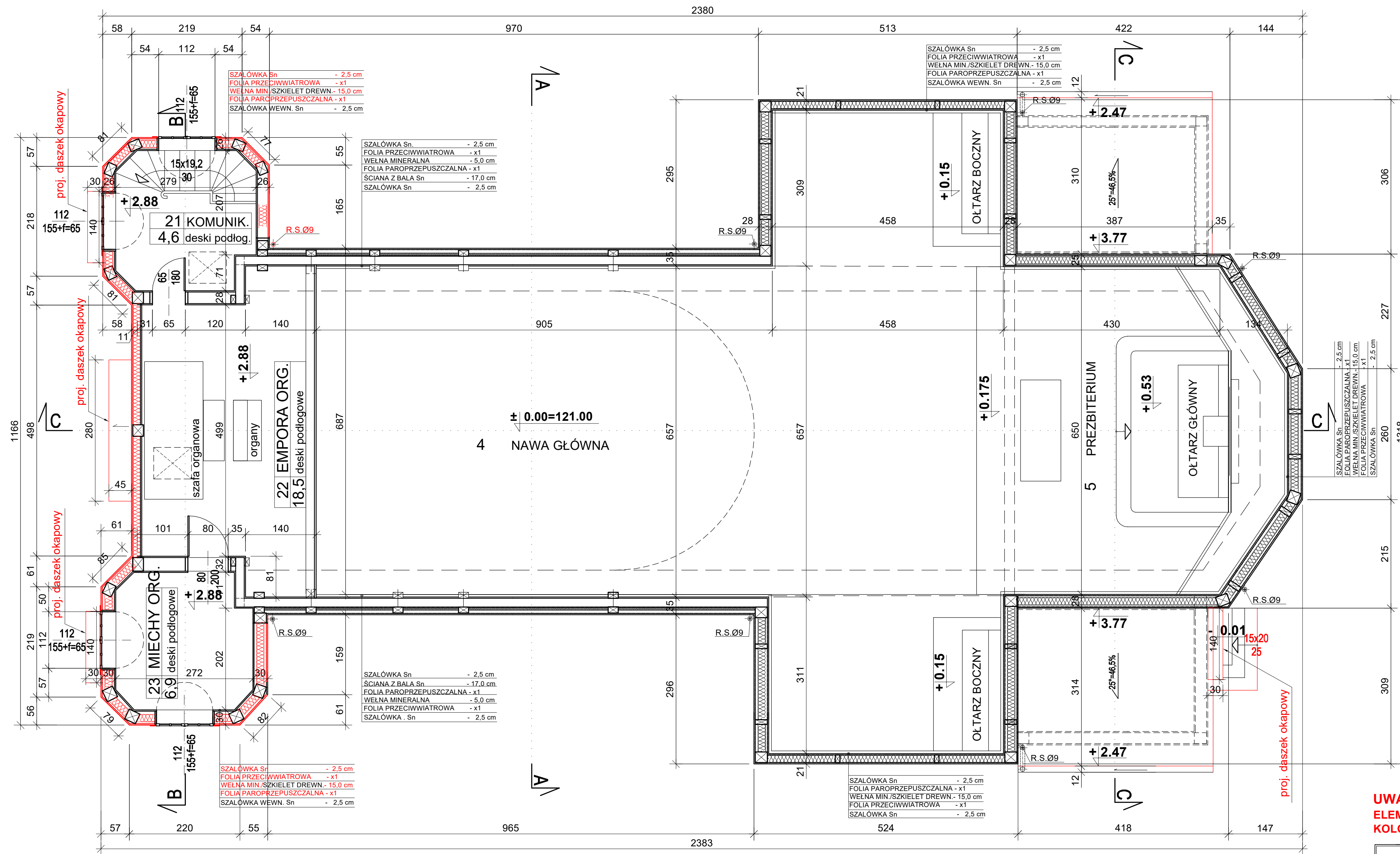
RZUT POZIOMU +4,00 1:50
