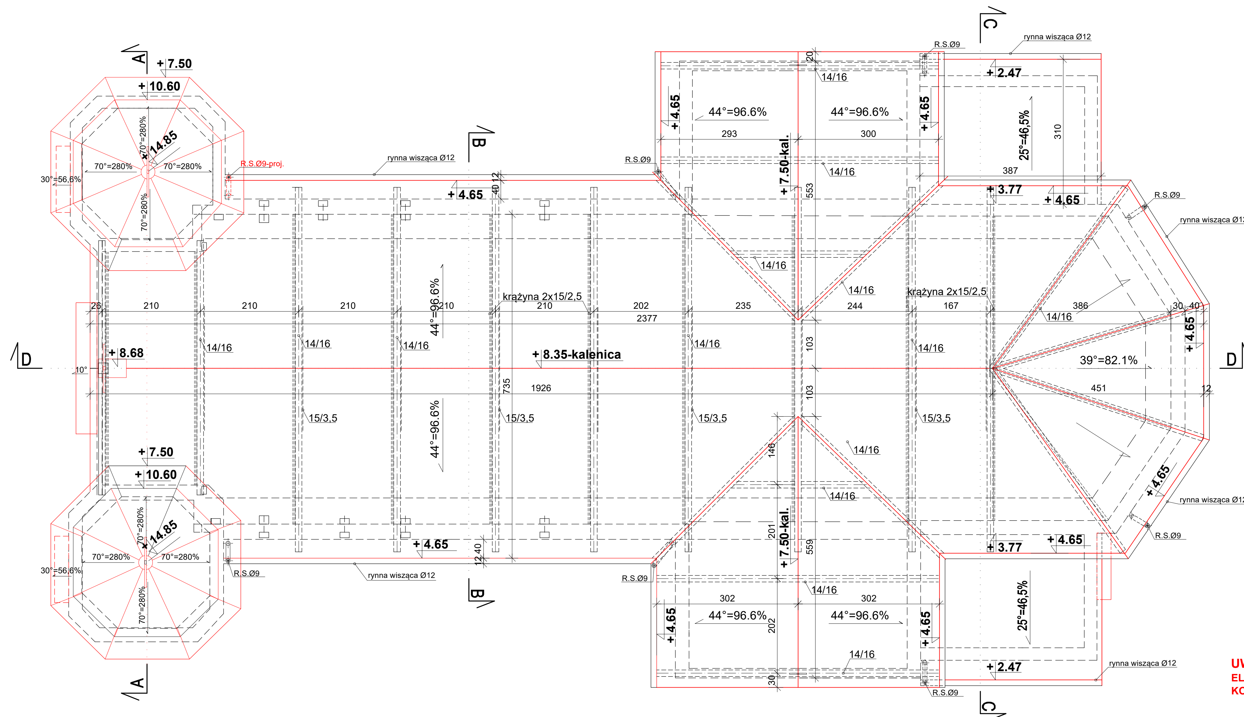
RZUT DACHU I WIĘŻBY 1:50
