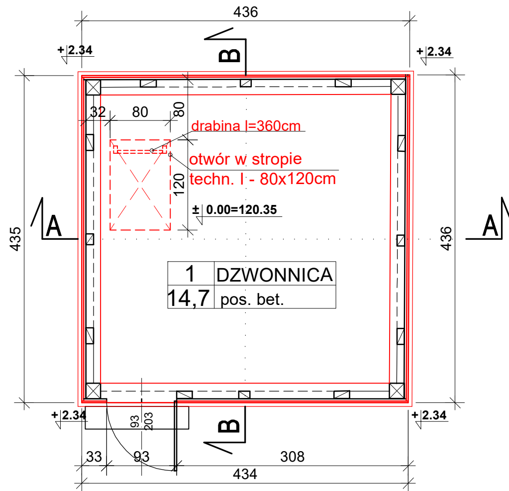
RZUT PRZYZIEMIA 1:50
