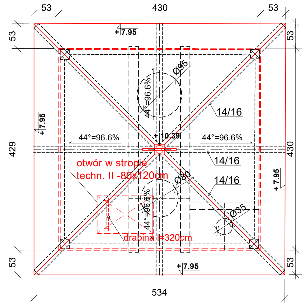
RZUT WIĘZBY I DACHU 1:50
